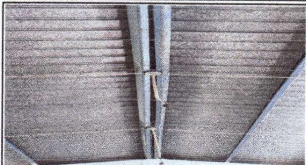
Foto1: Modulo aulas: el capote está con picaduras por el oxido, en union de laminas se filtra el agua
